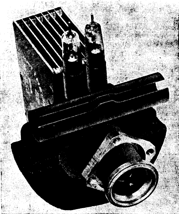
FIG. 19-14.—2J38 magnetron.
